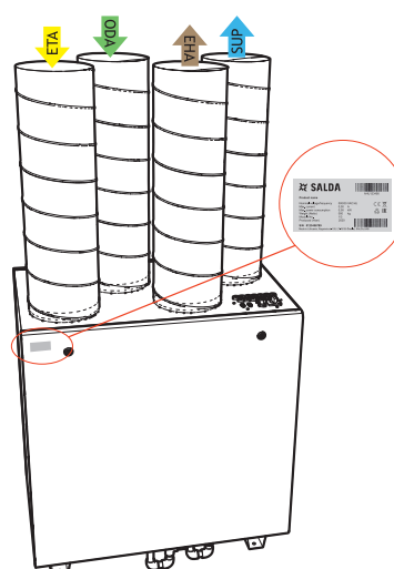
Rys. 2.4. Umieszczenie etykiety technicznej i oznaczenie króćców powietrza (left version)
