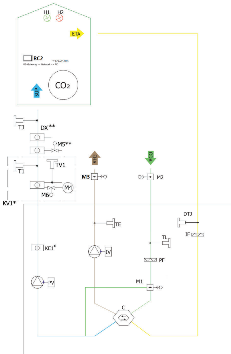
Rys. 5.1. * KE1 – tylko w wersji z nagrzewnicą elektryczną; * KV1 – stosowane w wersji z nagrzewnicą wodną; ** Możliwość sterowania.
