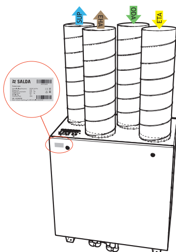
Rys. 2.3. Umieszczenie etykiety technicznej i oznaczenie króćców powietrza (right version)
