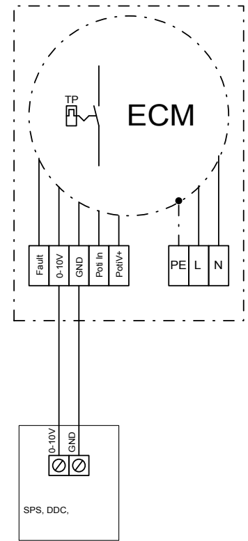
Przyłącze sygnału 0-10 V
